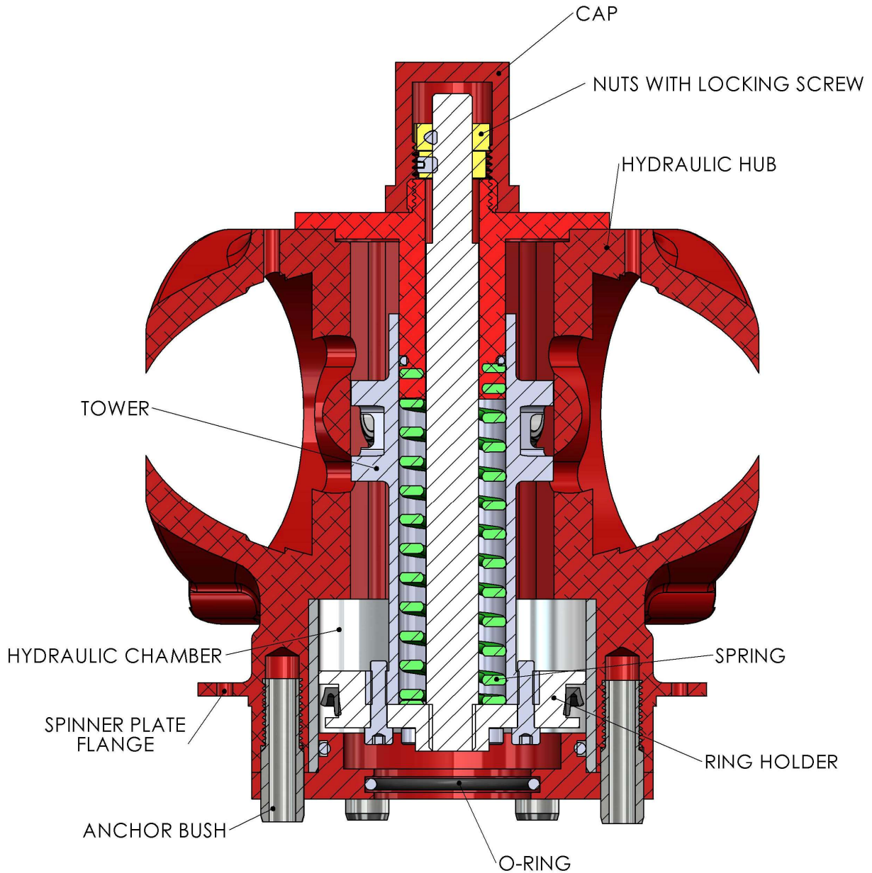
Fig. 3.2 AA SECTION
