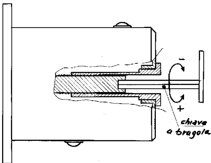
figura 21 regolazione manuale del passo, in caso di avaria elettrica.
